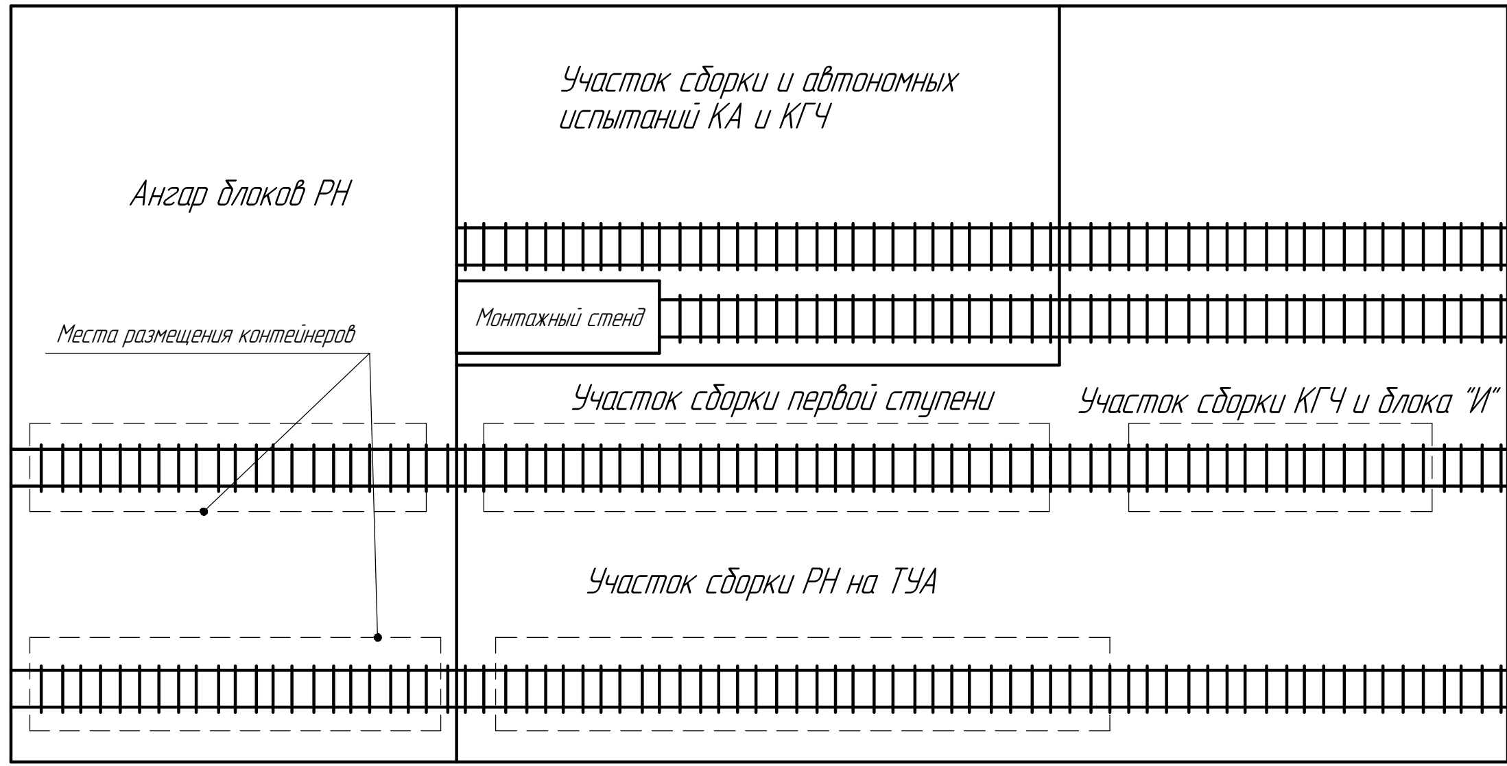
Схема монтажно-испытательного корпуса
